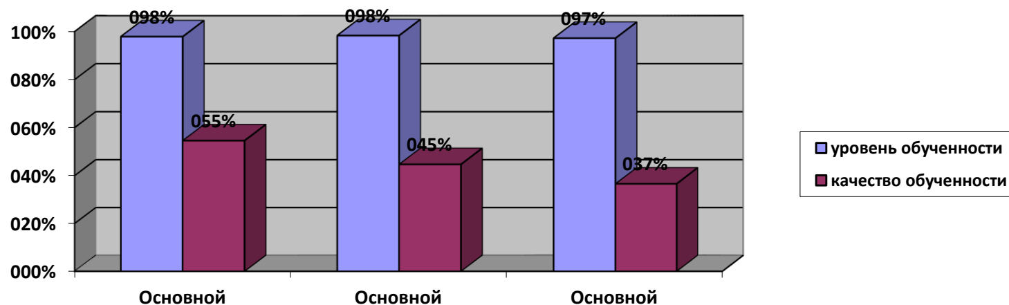
Динамика результатов ОГЭ по математике в Петрозаводском городском округе
